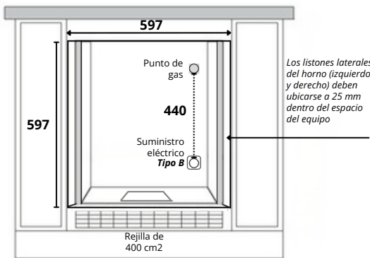
Diseño Traslapado Lateral (mm)
