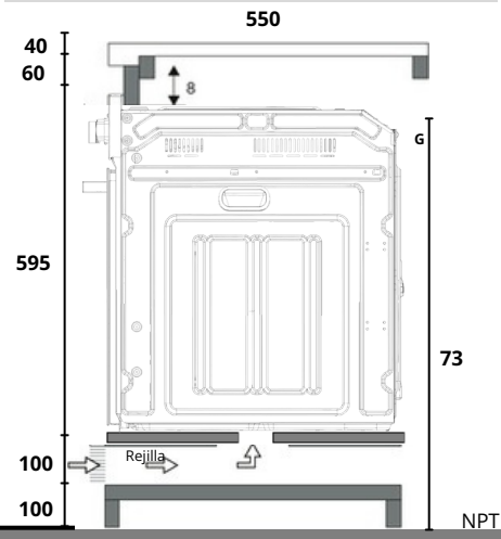
Diseño Traslapado Lateral (mm)
