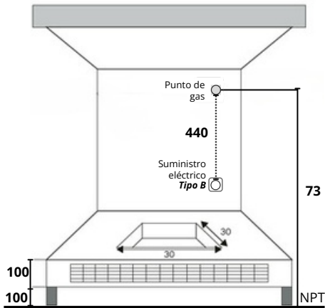
Diseño Traslapado Elevación (mm)
