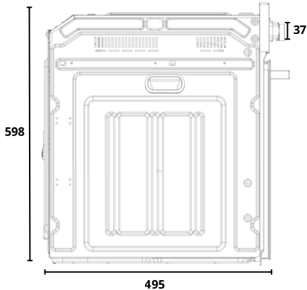
Ubicación Suministro (mm)
