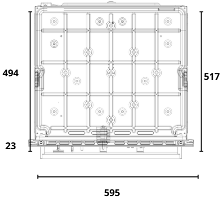
Diseño Embutido Elevación (mm)
