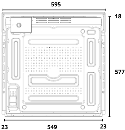
Vista Posterior (mm)
