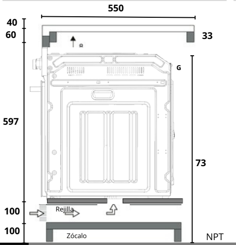
Diseño Embutido Lateral (mm)
